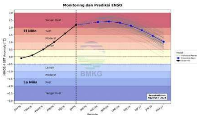
Gambar. 2.2.2 Prediksi ENSO
